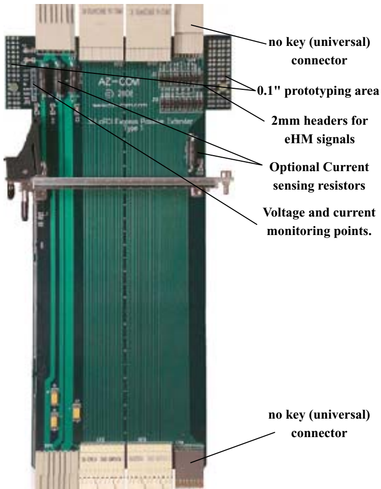
3U cPCIe Type1 Extender
